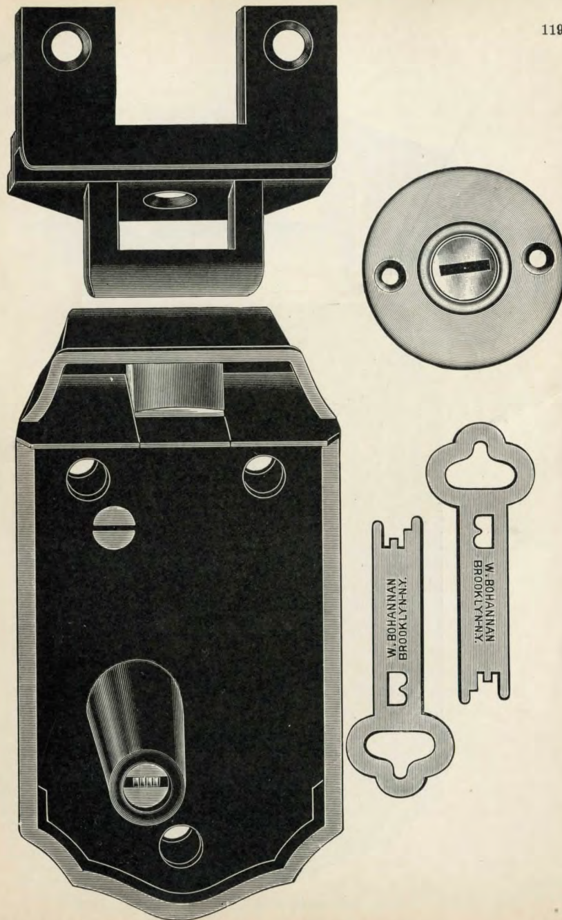
No. 213—Front. Plain Bevel Bolt.
